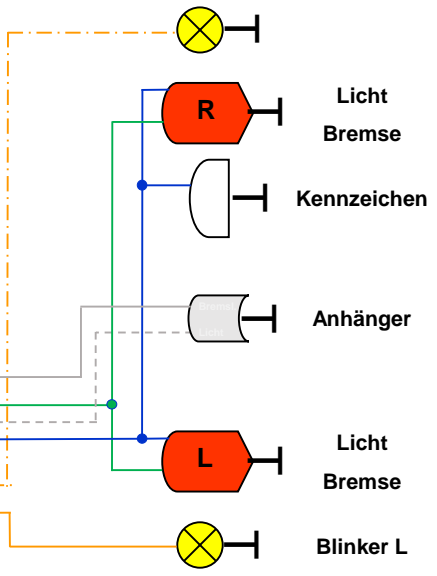
Schaltbild neu 12 Volt ohne Oldtimerschaltung
